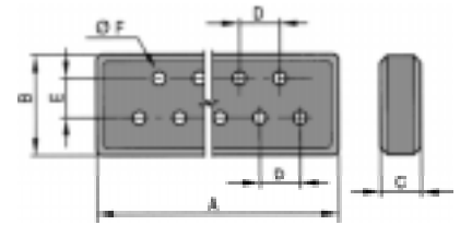
D - SUBPLATE
