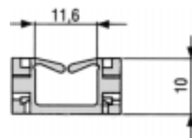
PROFIEL GESLOTEN ( CE )
