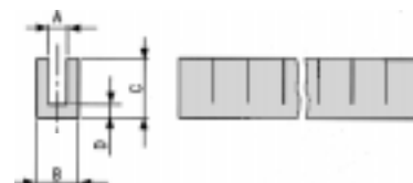
PROFIEL MET ZAAGSNEDEN ( CSG )
